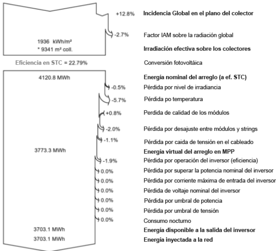
Diagrama 8. Pérdidas de un parque fotovoltaico de 250 kW de potencia de acople en la localidad de Hurlingham
