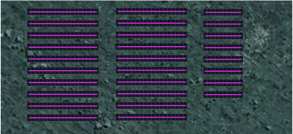
Diagrama 3. Layout propuesto para el parque de 250 kW en la localidad de General Daniel Cerri
