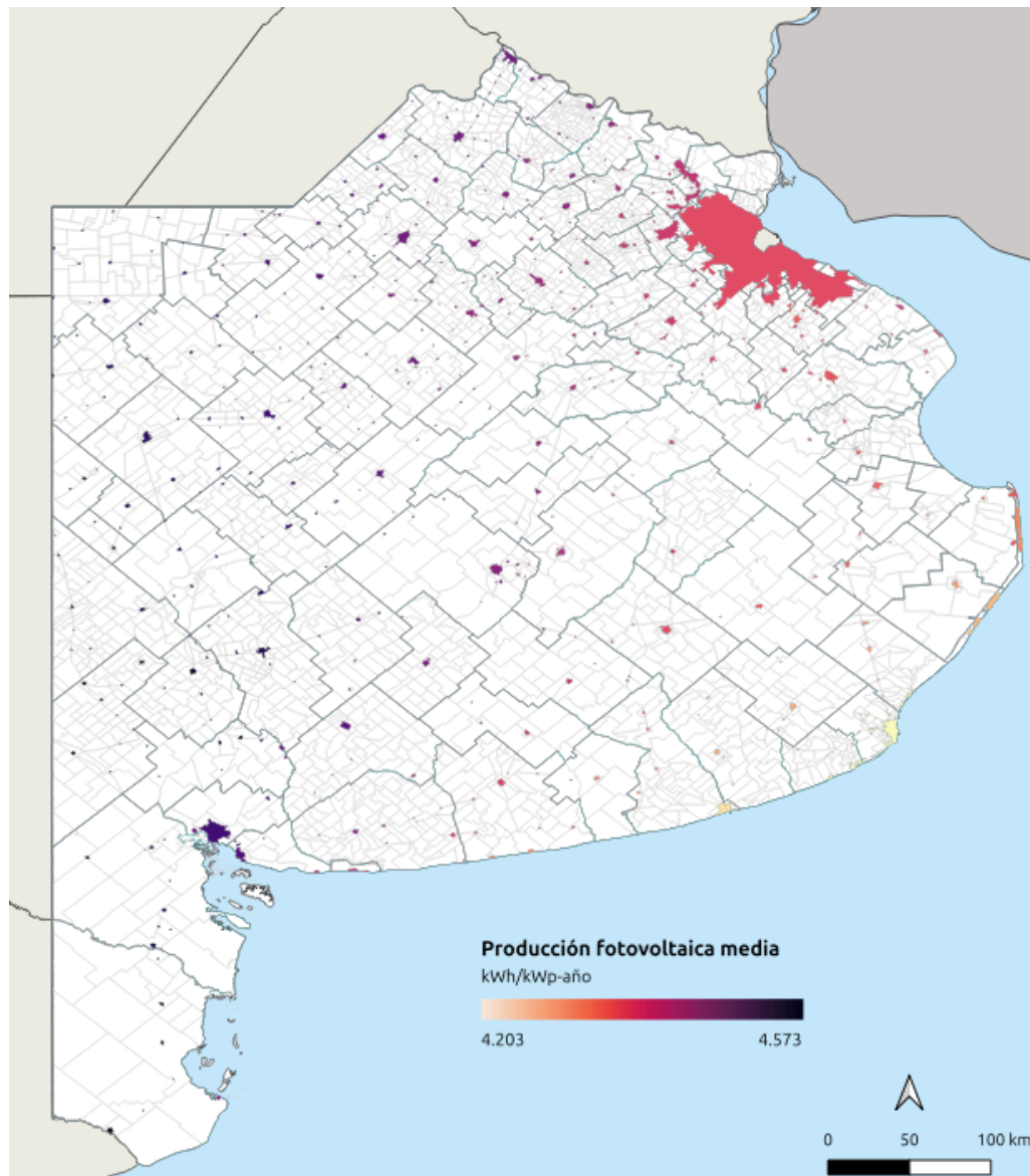
Mapa 9. Potencial de producción fotovoltaica media anual promedio para cada localidad (en kWh/kWp-año).
