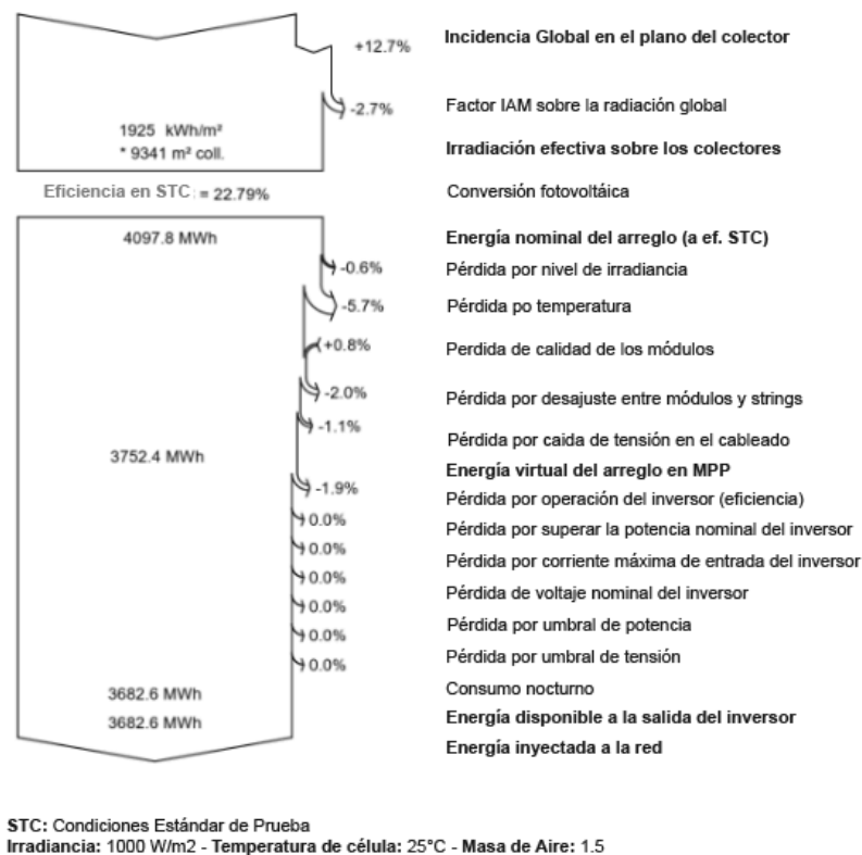
Diagrama 6. Pérdidas de un parque fotovoltaico de 250 kW de potencia de acople en la localidad de San Andrés de Giles
