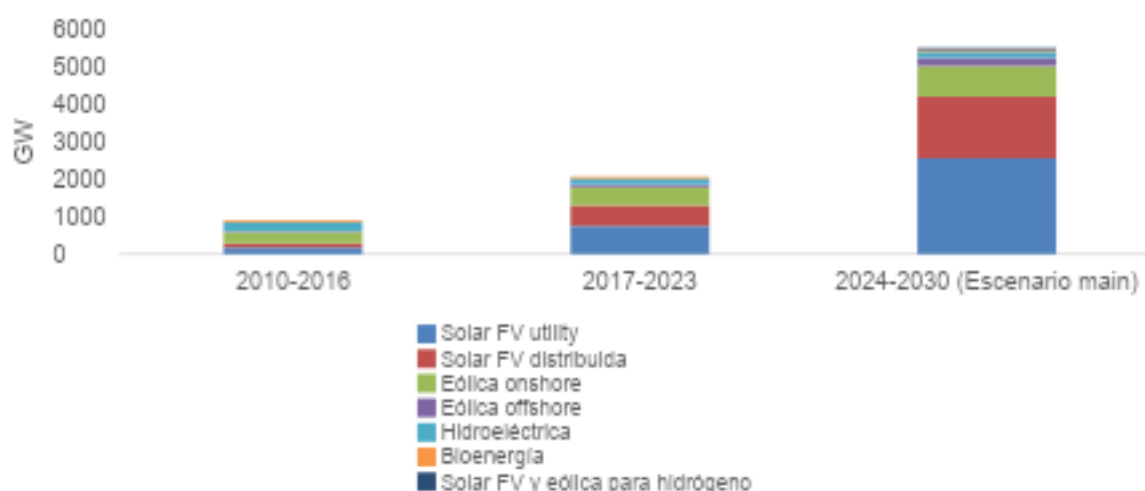
Gráfico 4. Crecimiento de la potencia renovable a nivel global por segmento tecnológico en GW (2010-2030)
