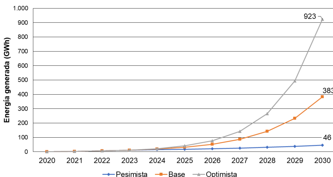
Gráfico 15. Generación anual de energía eléctrica proyectada a partir de GD (GWh)
