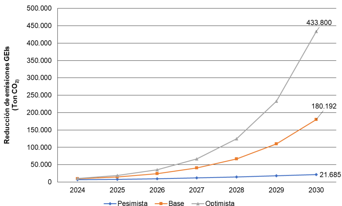
Gráfico 22. Reducción anual de emisiones de GEI por expansión de la potencia solar fotovoltaica en GD (ton CO 2 )
