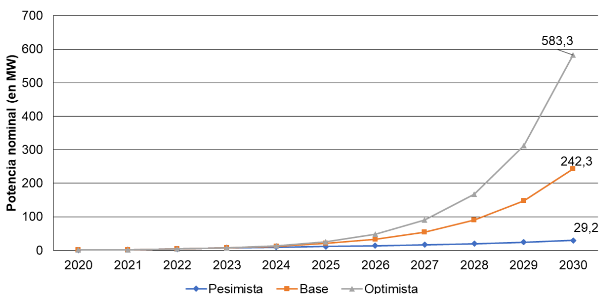
Gráfico 14. Proyección de potencia nominal de generación solar fotovoltaica a instalar de GD en PBA (en MW)
