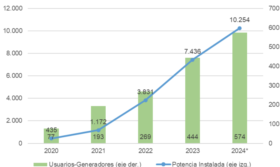
Gráfico 11. Potencia instalada (kW) y cantidad de UG de GD en la Provincia de Buenos Aires (período 2020-2024).
