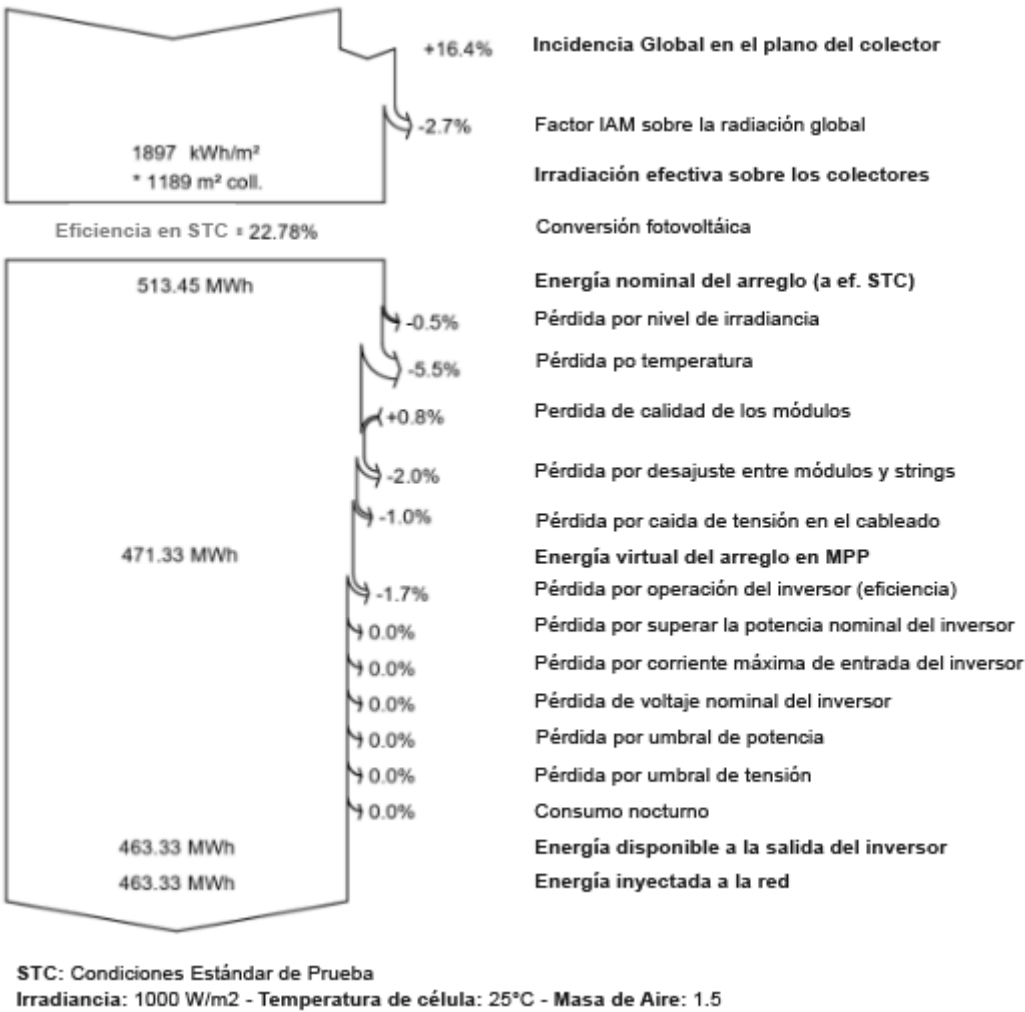
Diagrama 4. Pérdidas de un parque fotovoltaico de 250 kW de potencia de acople en la localidad de General Daniel Cerri
