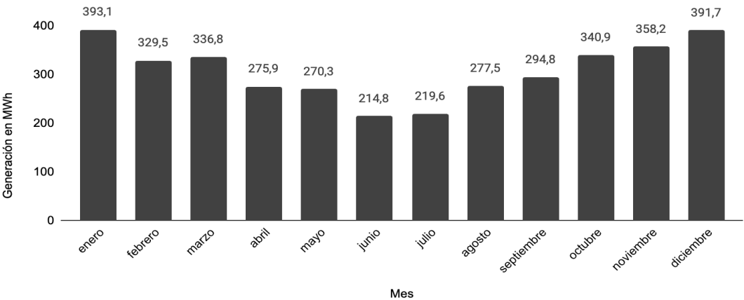
Gráfico 26. Generación mensual estimada para el parque de la localidad de Hurlingham (en MWh)
