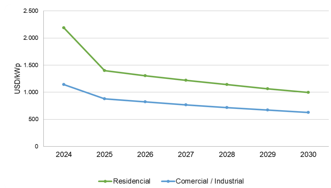
Gráfico 16. Evolución del valor de la inversión de capital en instalaciones de GD para Argentina (USD/kWp)
