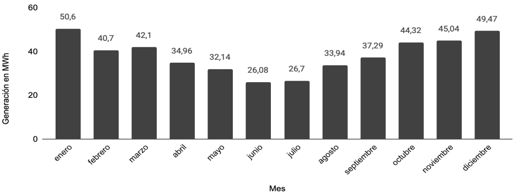
Gráfico 24. Generación mensual estimada para el parque de la localidad de General Daniel Cerri (en MWh)
