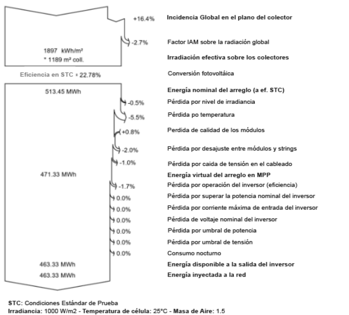
Diagrama 2. Pérdidas de un parque fotovoltaico de 250 kW de potencia de acople en la localidad de Merlo
