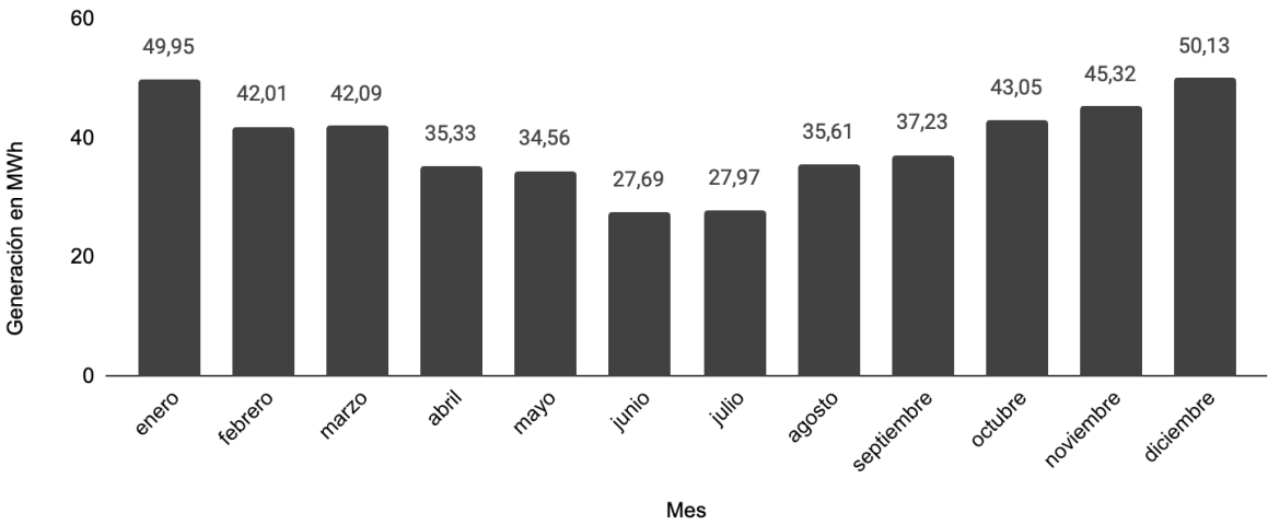
Gráfico 23. Generación mensual estimada para el parque de la localidad de Merlo (en MWh)
