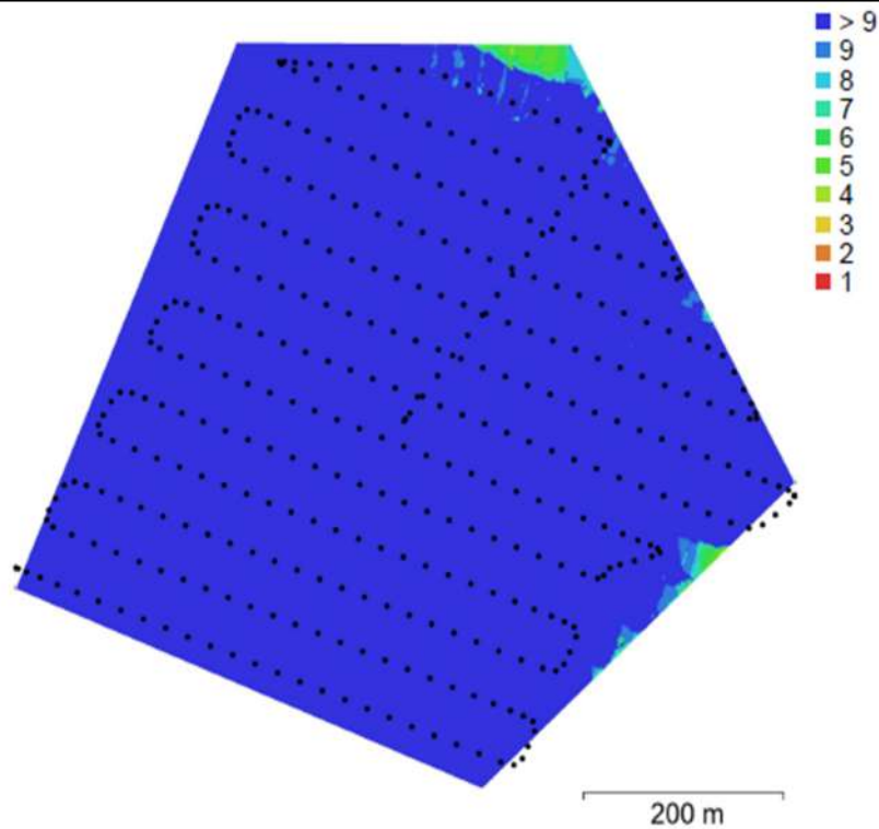
Fig. 1. Posiciones de cámaras y solapamiento de imágenes.
