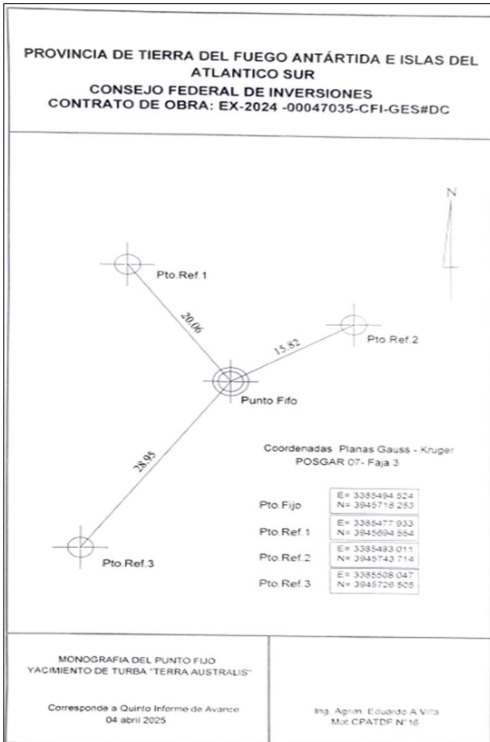
Figura 33. Monografía de punto fijo. Yacimiento Terra Australis, 2025.
