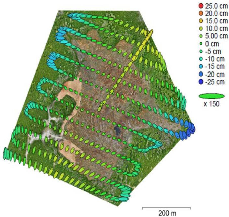
Fig. 3. Posiciones de cámaras y estimadores de error.
