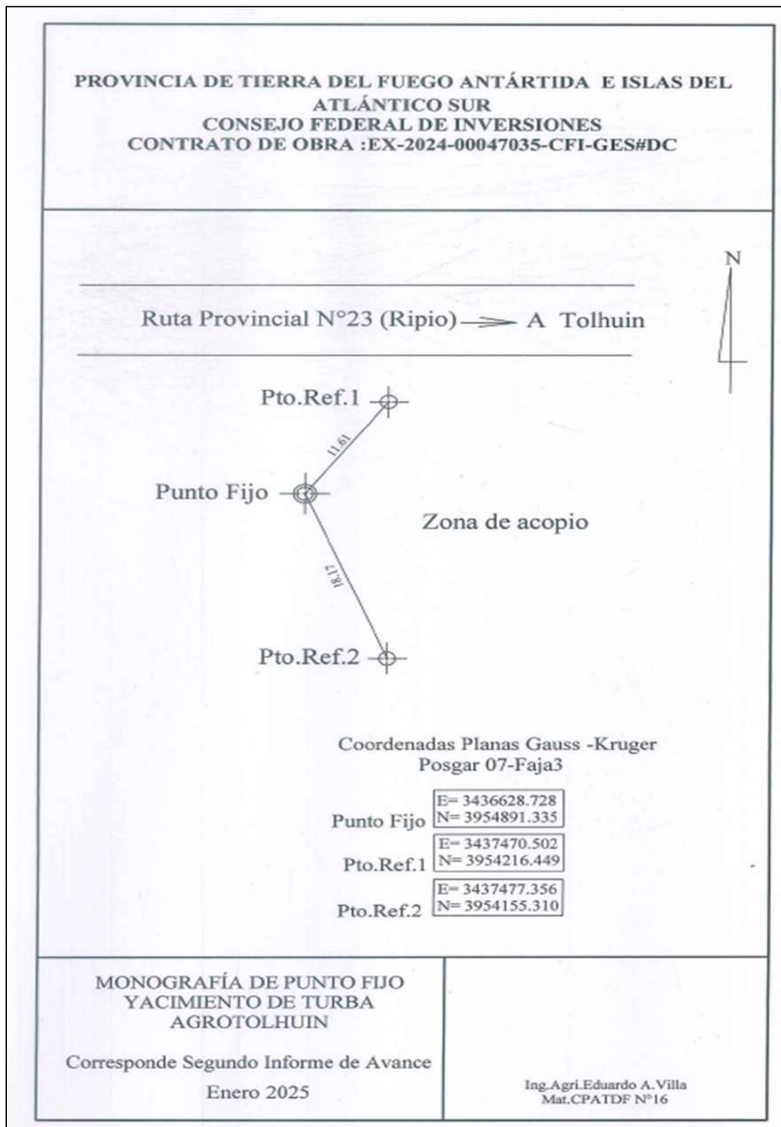
Figura 11. Monografía de punto fijo. Yacimiento Agrotolhuin, 2025.
