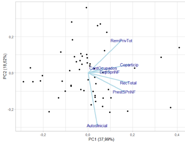
Figura 9. Biplot (valores individuales y variables)
