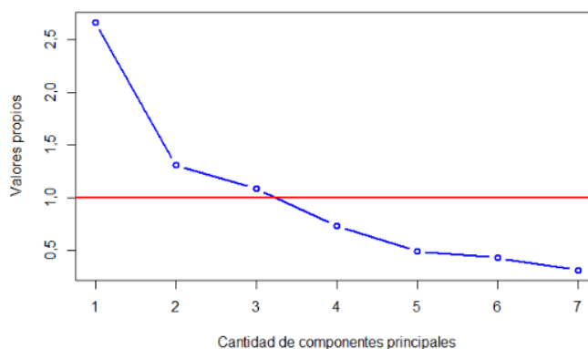
Figura 10. Scree Plot (valores propios ordenados vs. cantidad de componentes principales)
