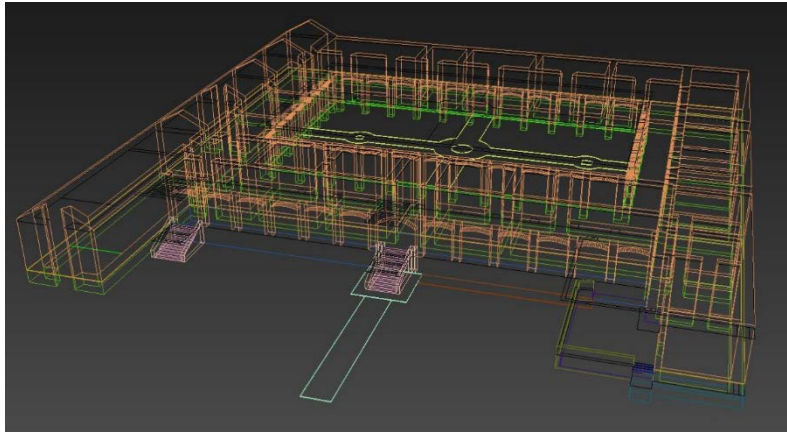
Imagen 2. Primeros bosquejos del relevamiento arquitectónico.
