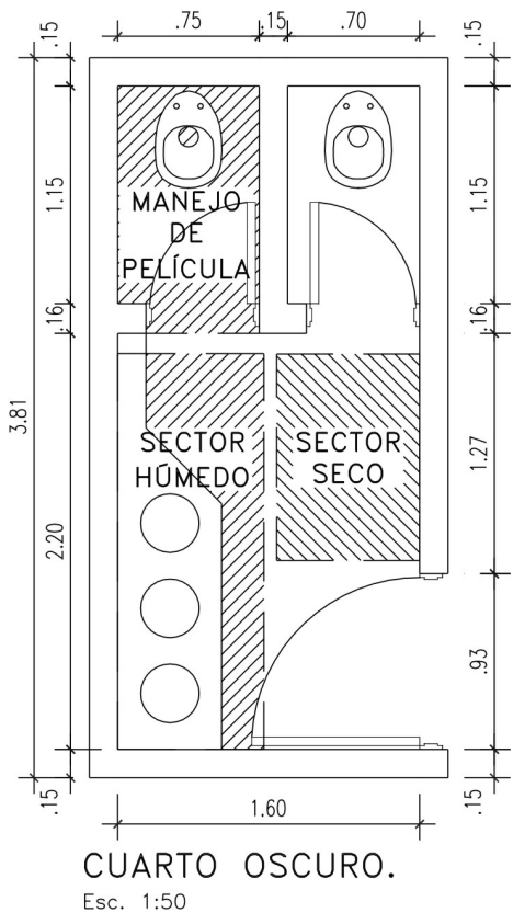
Planta esquemática e indicación de áreas del cuarto oscuro.
