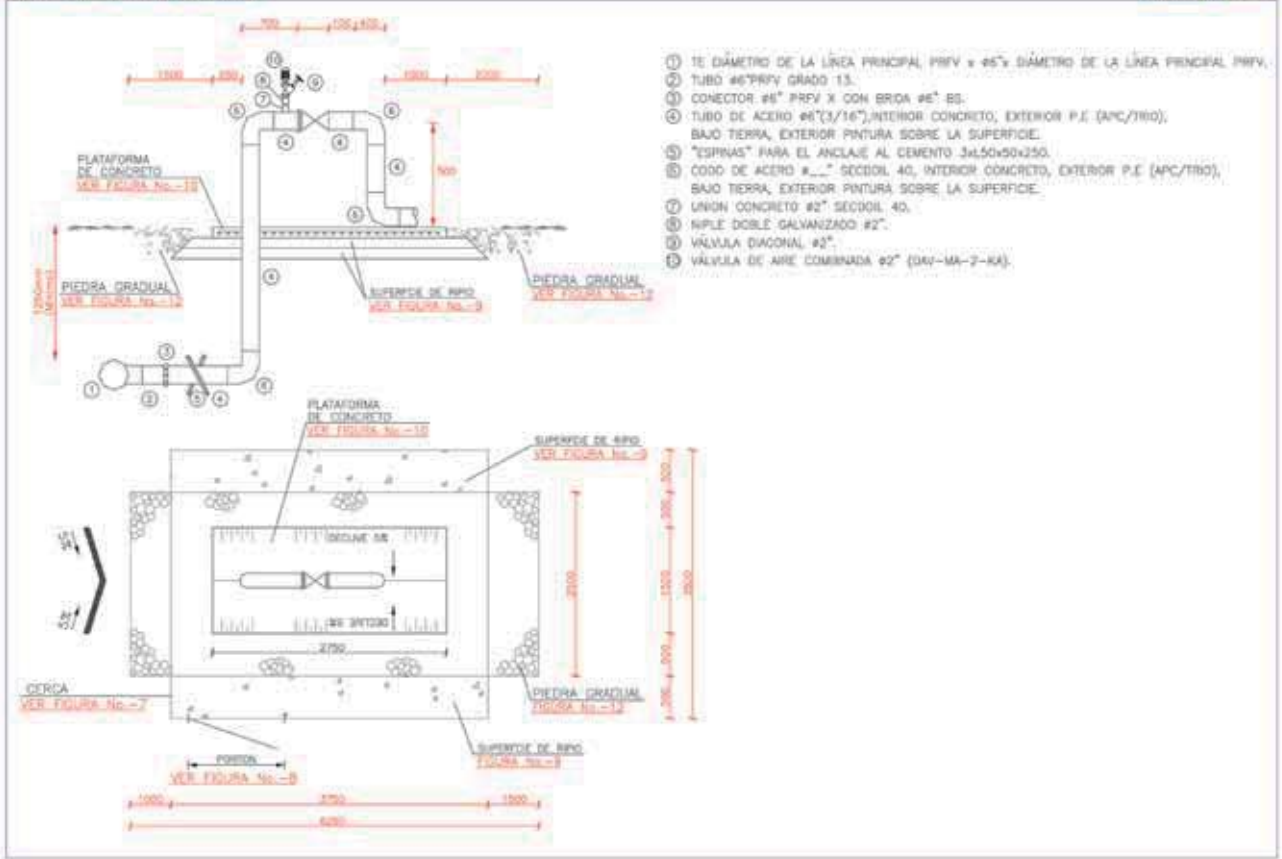
FIGURA DE DRENAJE EN LÍNEA
