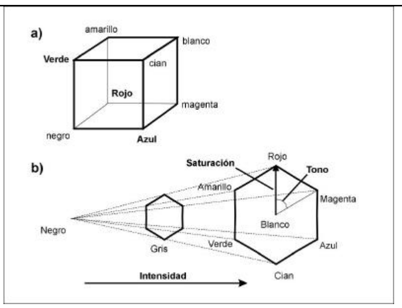
Figura 5. Representación gráfica de las coordenadas de color en los espacios: a) RGB (cubo) b) HSI (hexacono).
