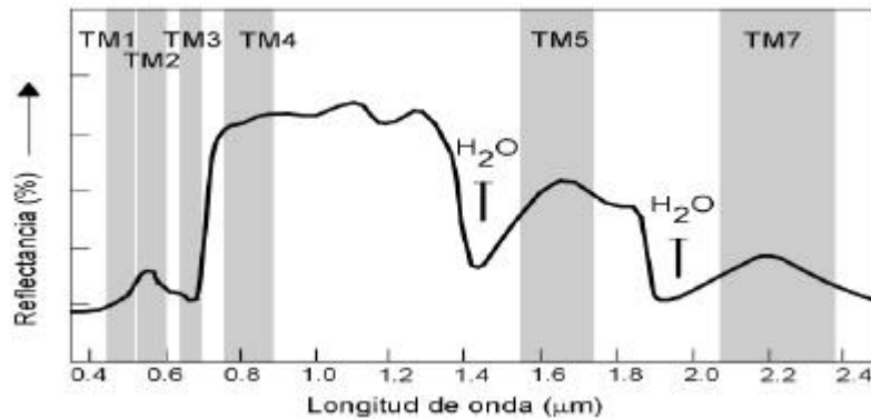
Figura 7. Firma espectral característica de la vegetación sana en comparación con los intervalos espectrales de las imágenes LANDSAT-TM y ETM +
