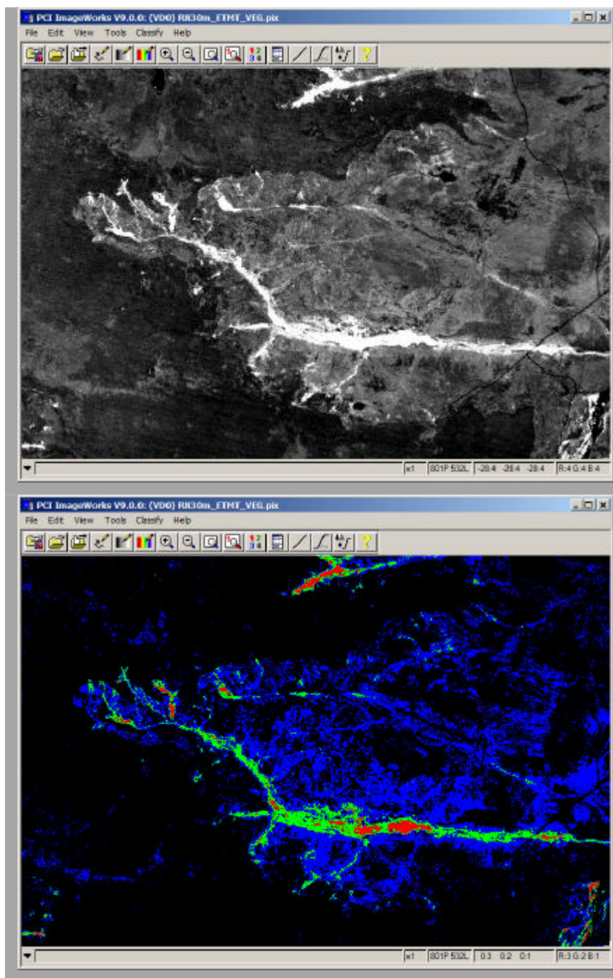
Figura 8. Imágenes tendientes a realzar la presencia de vegetación: Imagen de Índice de Vegetación (arriba) y resultado de la segmentación de densidades (abajo).
