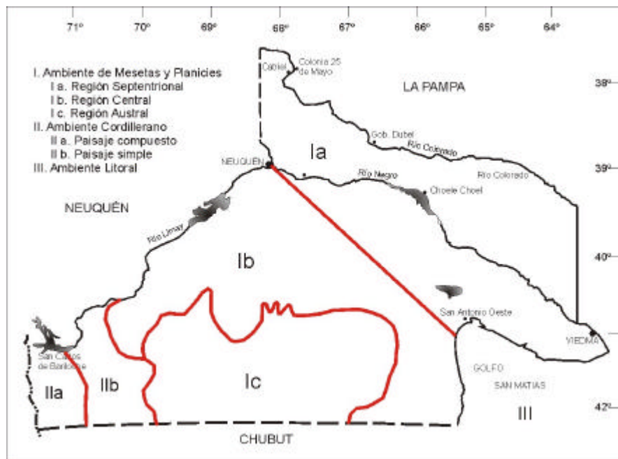
Figura 15. Ambientes y rasgos geomorfológicos de la provincia de Río Negro. (Extraído de González Díaz y Malagnino, 1984.)
