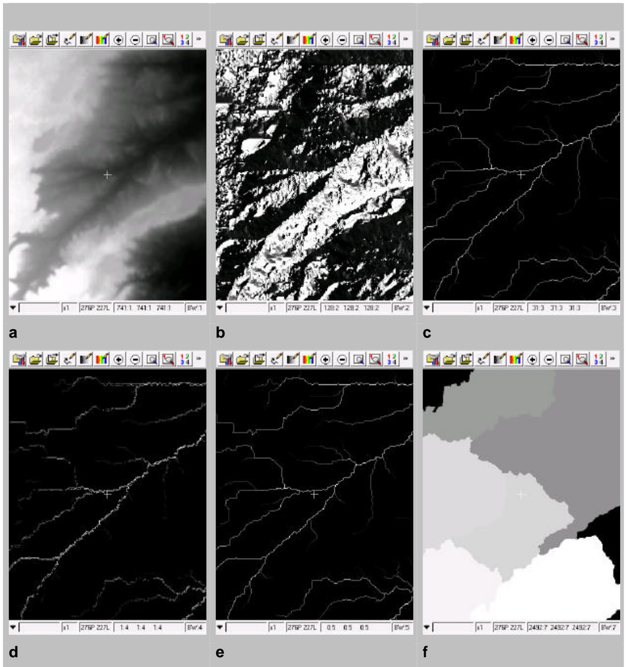
Figura 14. Pasos seguidos para la extracción semi-automática de redes de drenaje y divisorias de cuencas a partir del DEM del Shuttle: a) rellenado de depresiones, b) direcciones de flujo, c) acumulación de flujo, d) valor delta de flujo, e) red de drenaje (umbral n=1000 ), f) cuencas hidrográficas (umbral n=10000 ).
