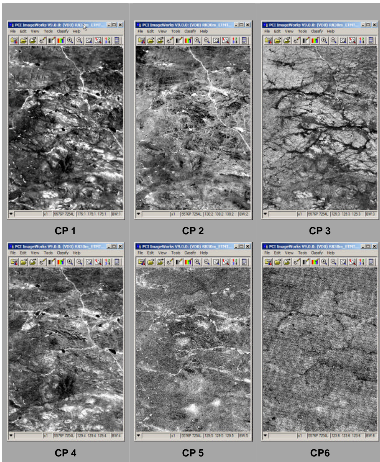
Figura 10. Imágenes de componentes principales para un sector del área de estudio.
