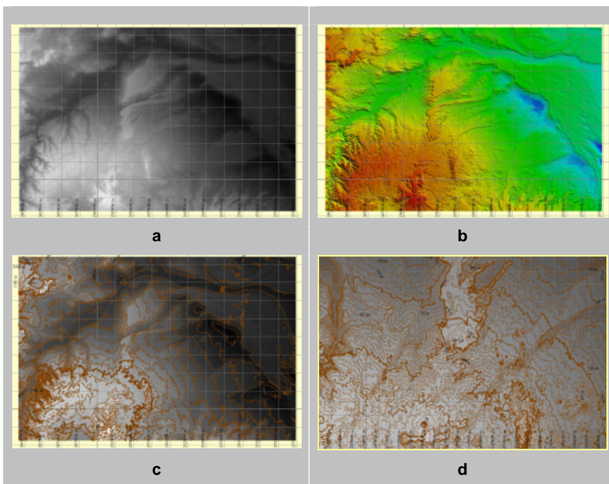
Figura 13. Modelo Digital de Elevación a) en niveles de gris y b) en pseudocolor, c) con las curvas de nivel superpuestas (100 m), d) detalle del anterior (25 m).
