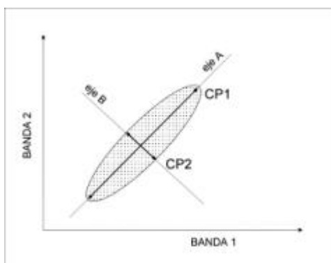
Figura 9. Obtención de Componentes Principales a partir de 2 bandas espectrales.
