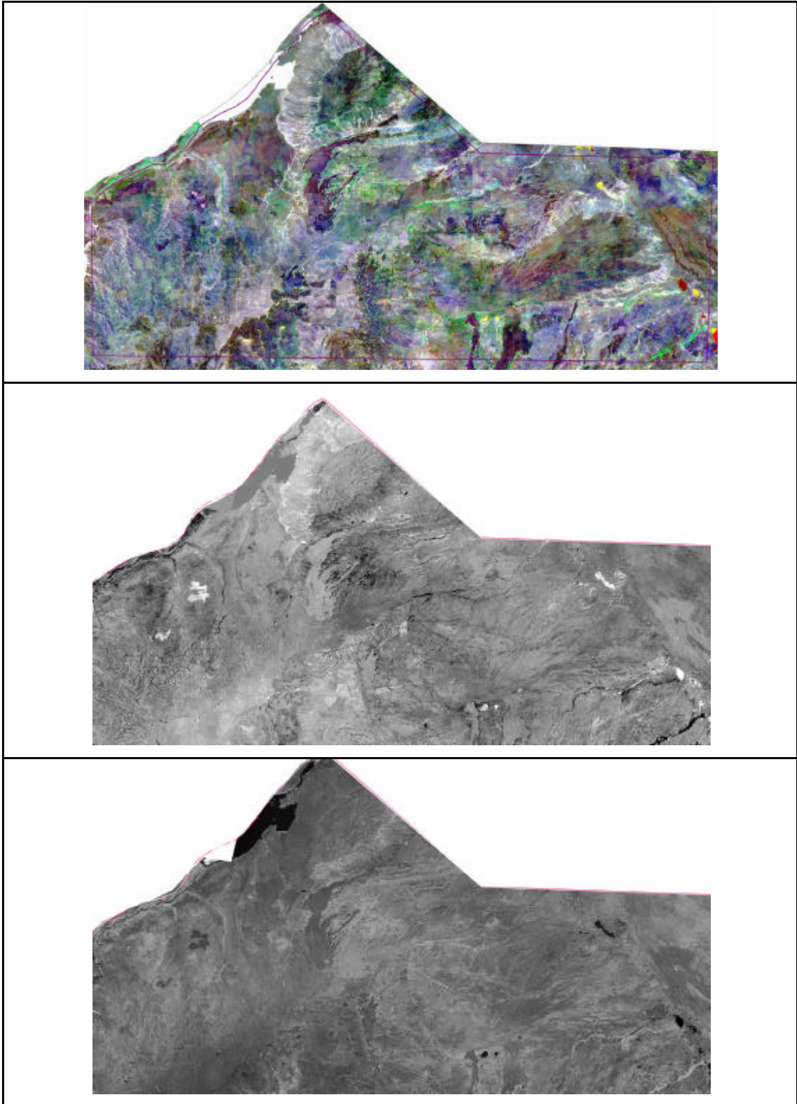
Figura 11. Imágenes RGB 543, ACP (componente PC3) y Índice de Vegetación
